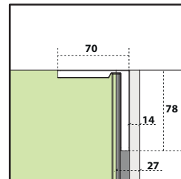
KLAMRA WEWNĘTRZNA
