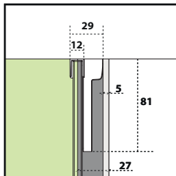
KLAMRA ZEWNĘTRZNA
