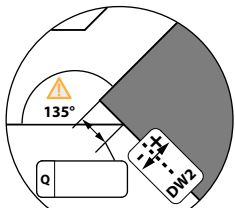
SZCZEGÓŁ A
