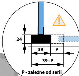
SZCZEGÓŁ A **
